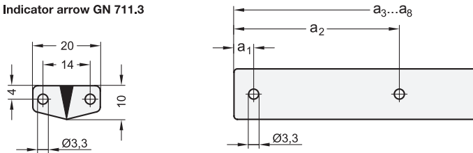
Indicator arrow GN 711.3
